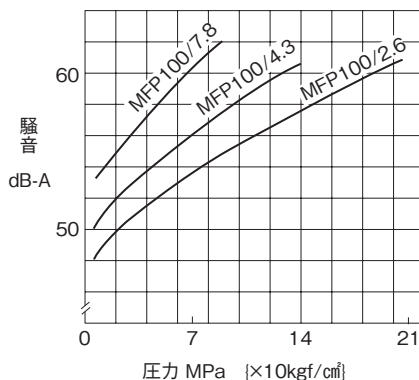
電動機1.5kW
