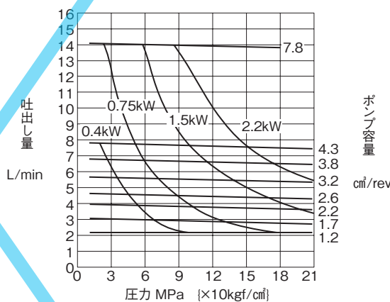
入力回転数：1800min -1
