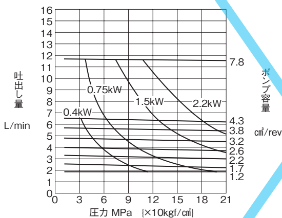
入力回転数：1500min -1
