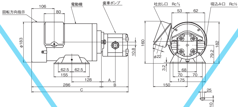
寸法表
