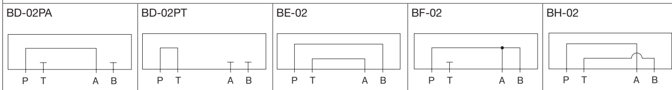
JIS油圧図記号
