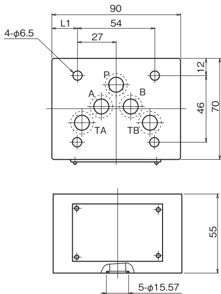
■寸法表
